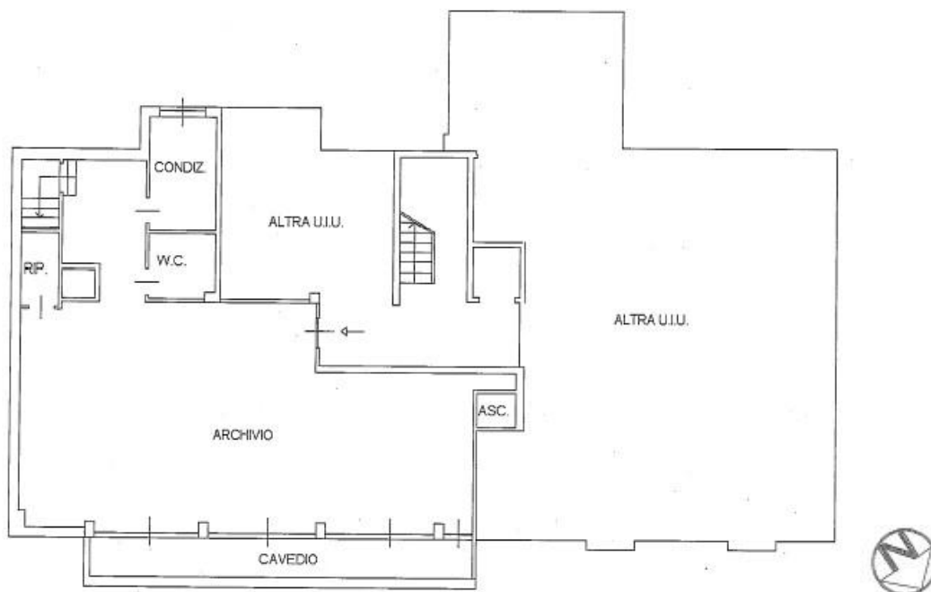
Planimetria catastale, non in scala, piano seminterrato
